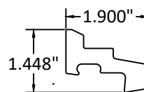
11B GLAZING BEAD - MONO. LAMI. PVC
