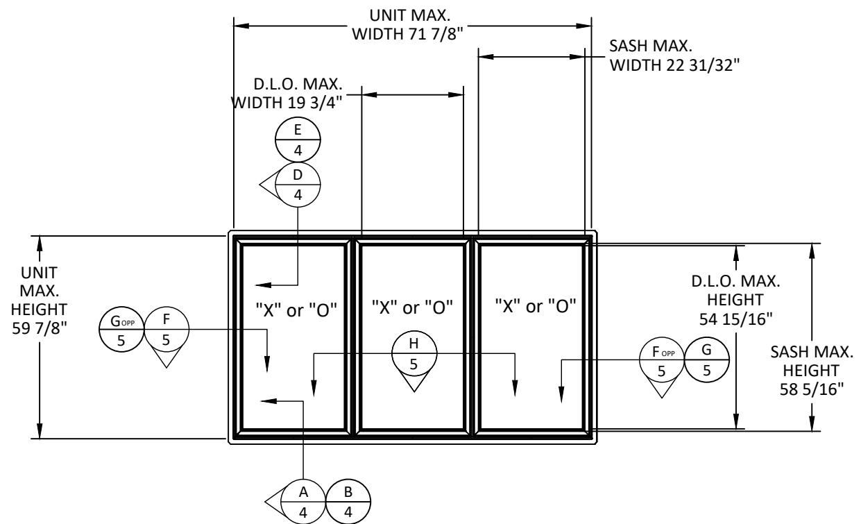
ELEVATION C35
