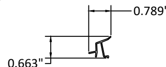
11B GLAZING BEAD - MONO. LAMI. PVC
